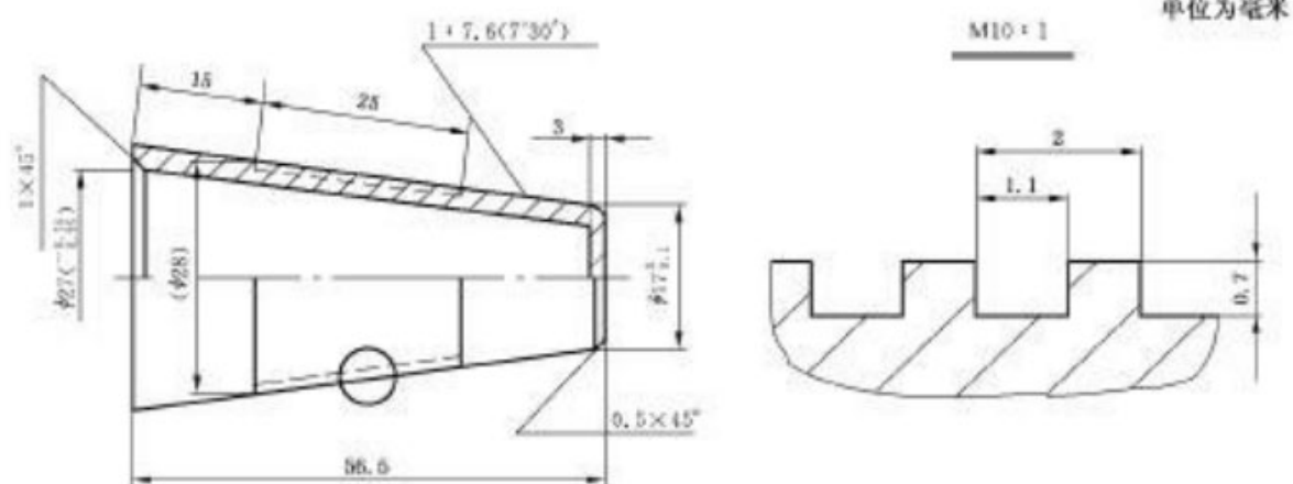
图 5 量热计内衬
